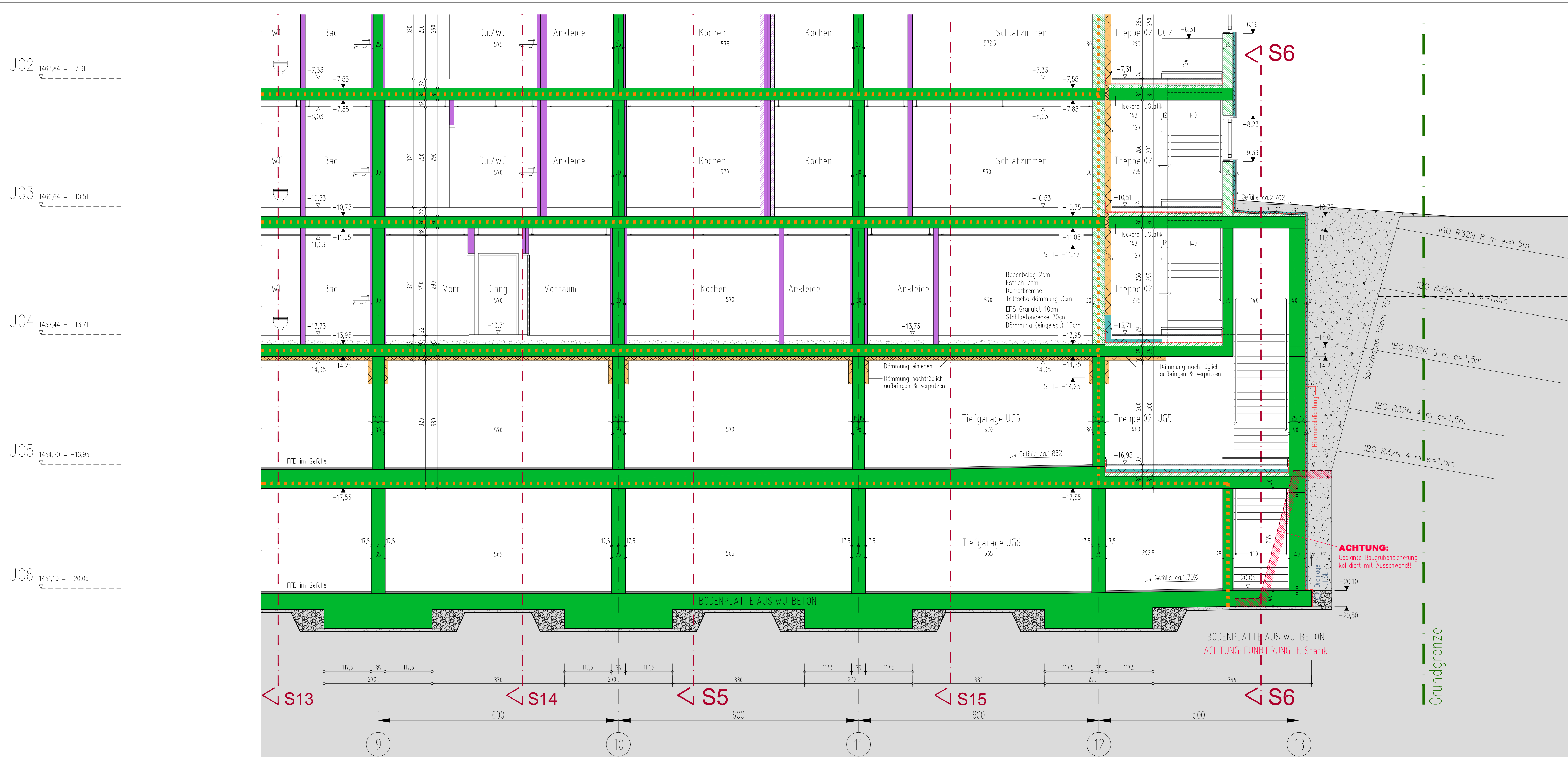
SCHNITT S7 - 1:50
